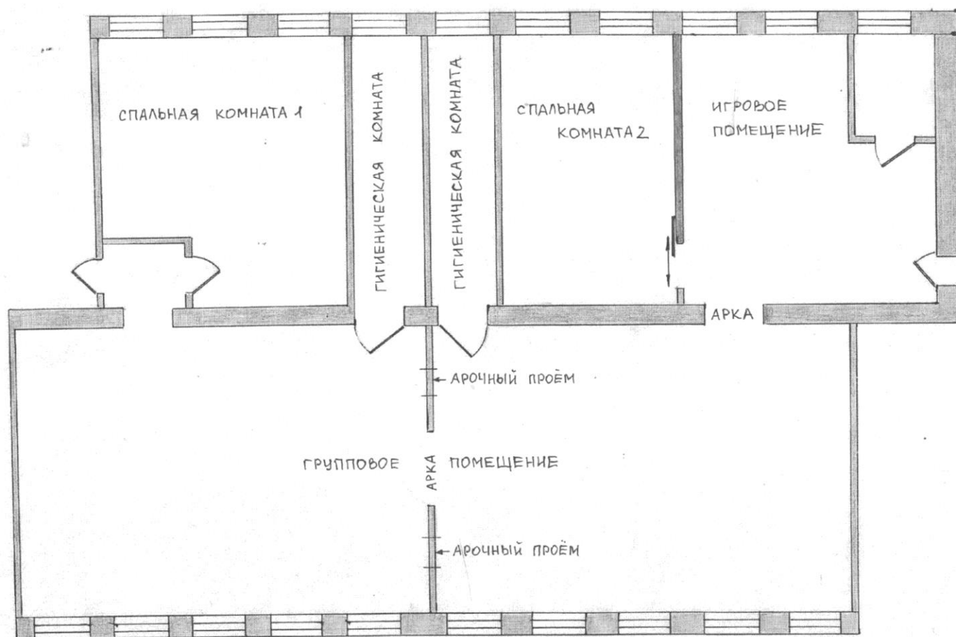
Рисунок 3. Планировка помещения группы №3 после реконструкции
